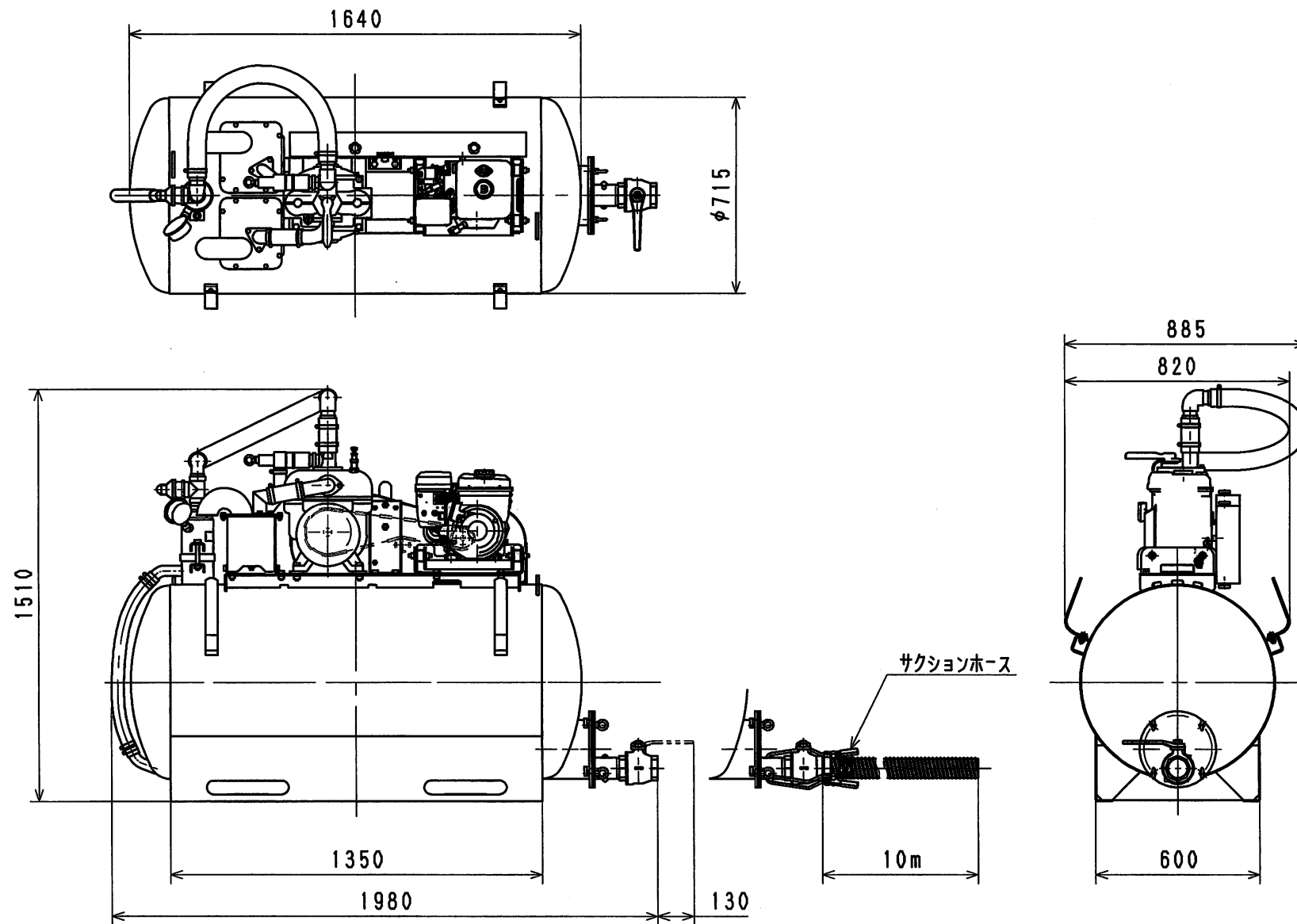
DV-605B バキュームカー外観図
