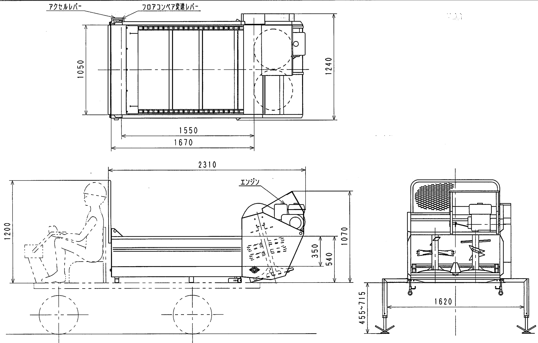
DM-620BN 外観図
