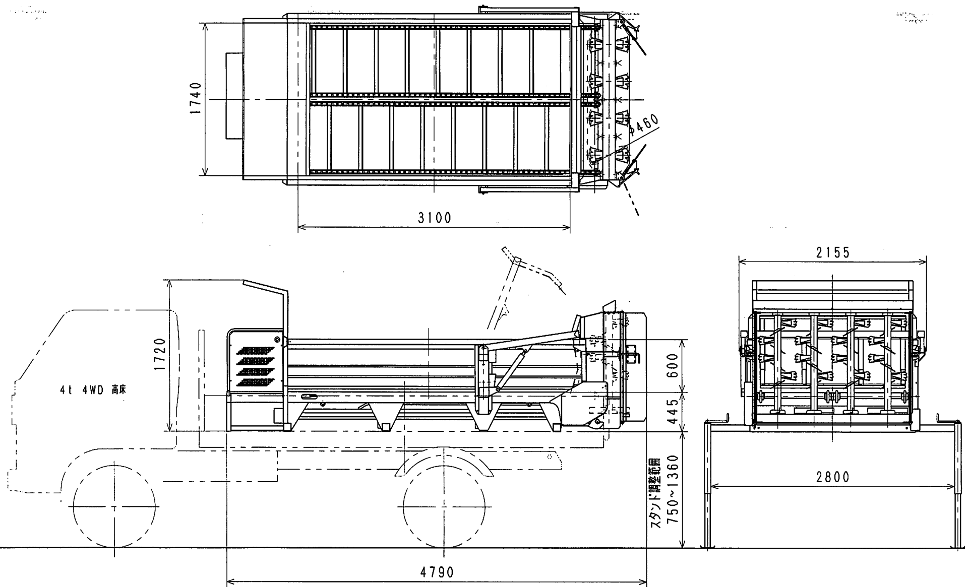
DM-3020BN マニアスフ° レッタ° 外観図
