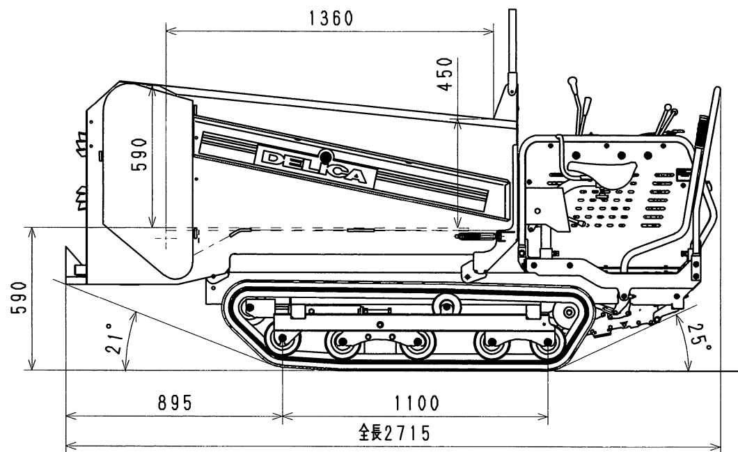
DAM-66T 自走マニアスプレッダ 外観図
