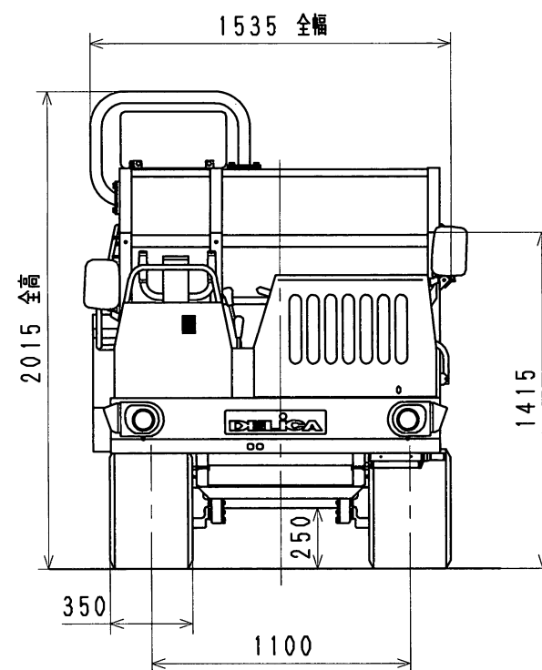
DAM-186Y 自走マニアスプレッダ 外観図
