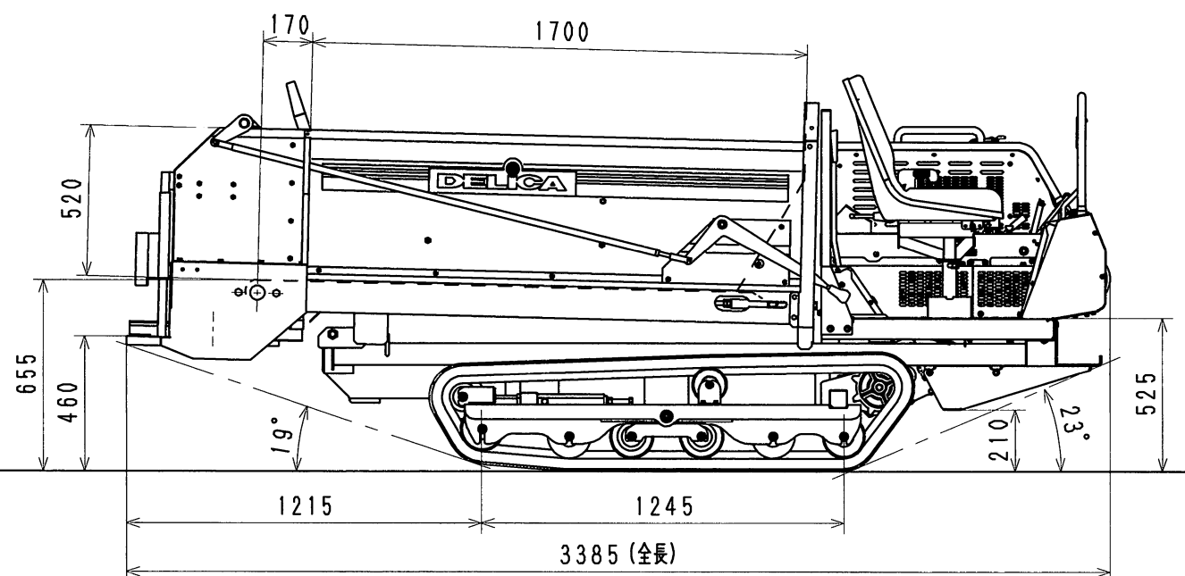
DAM-102S 自走マニアスプレッダ 外観図 1480300000
