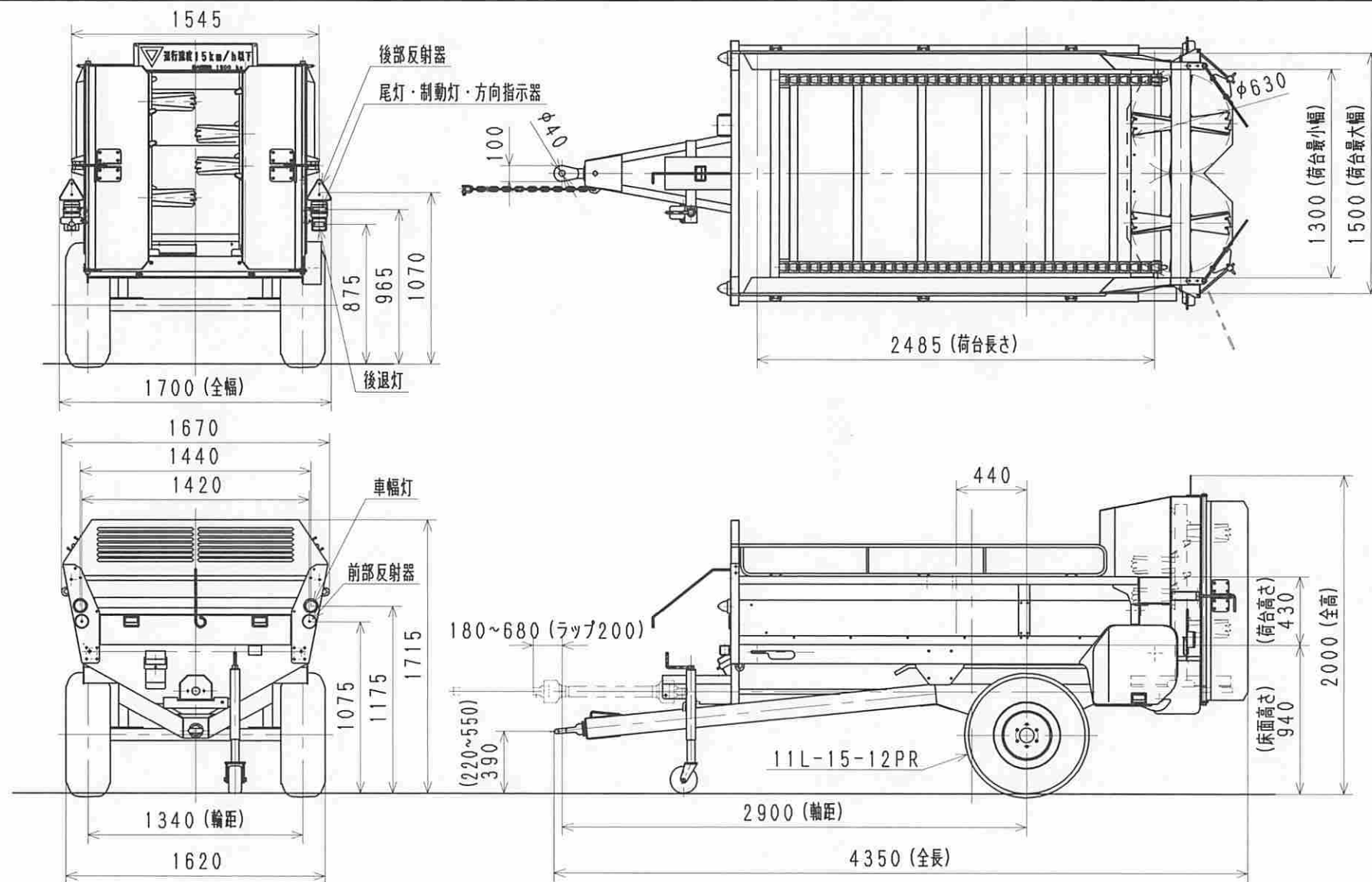
DXT-1525 マニアスプレッダ外観図
