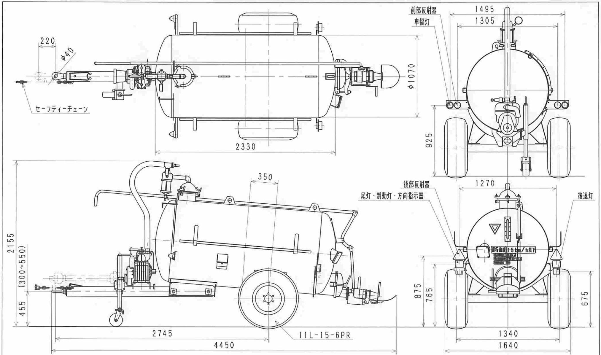
DV-1905T 外觀三面図
