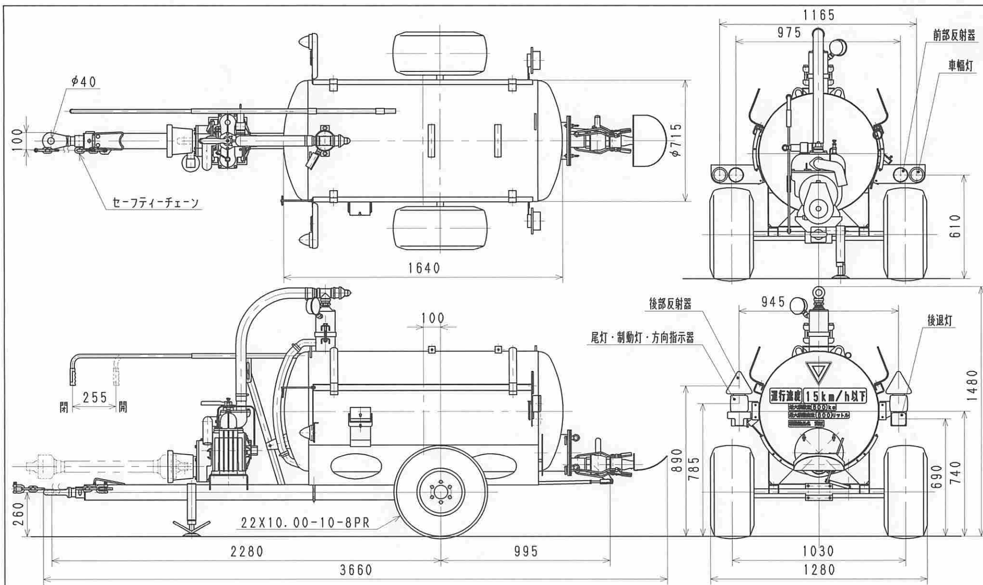
DV-605T バキュームカー-外觀図
