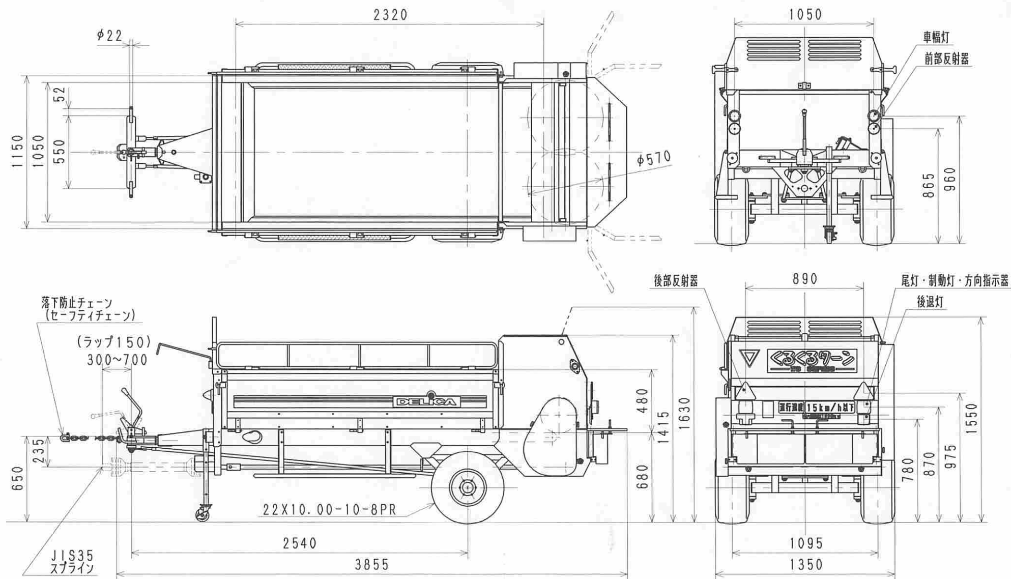
DMS-1105WS けん引マルチスプレッダ 外観図
