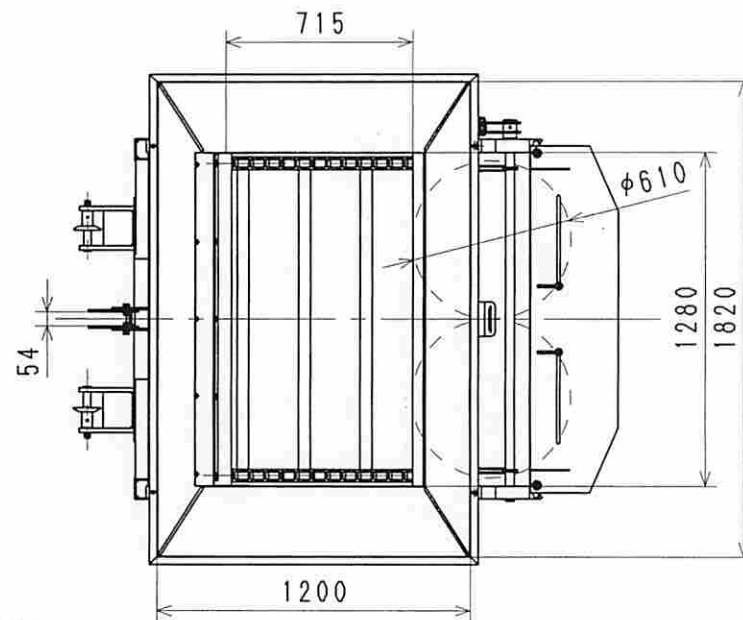
前部反射器
