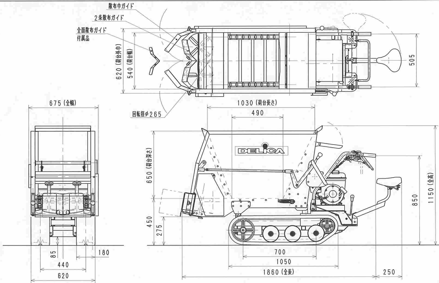
DAM-18SN 自走マルチスプレッダ 外観図
