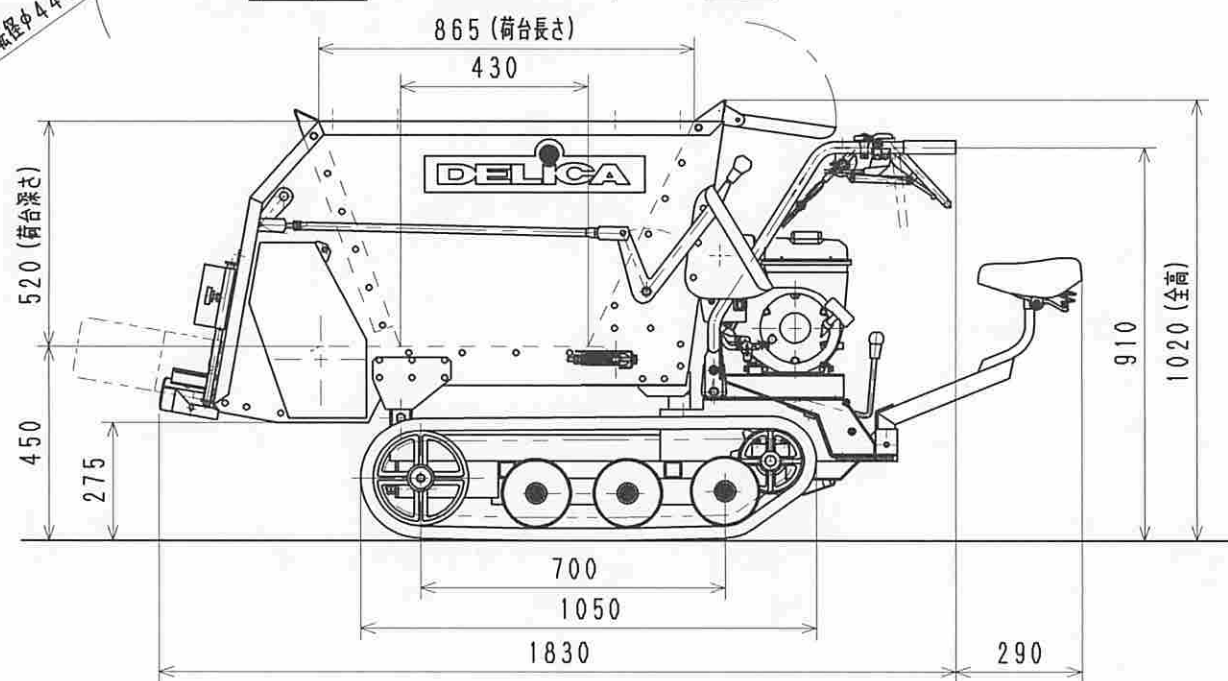
DAM-22SN 自走マルチスプレッド 外観図
