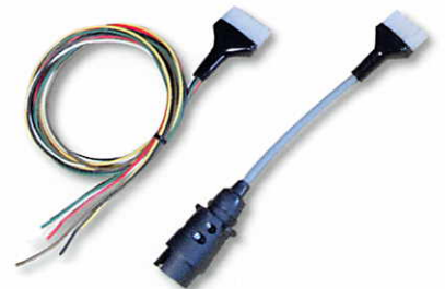
トラクタ側 変換ハーネス
