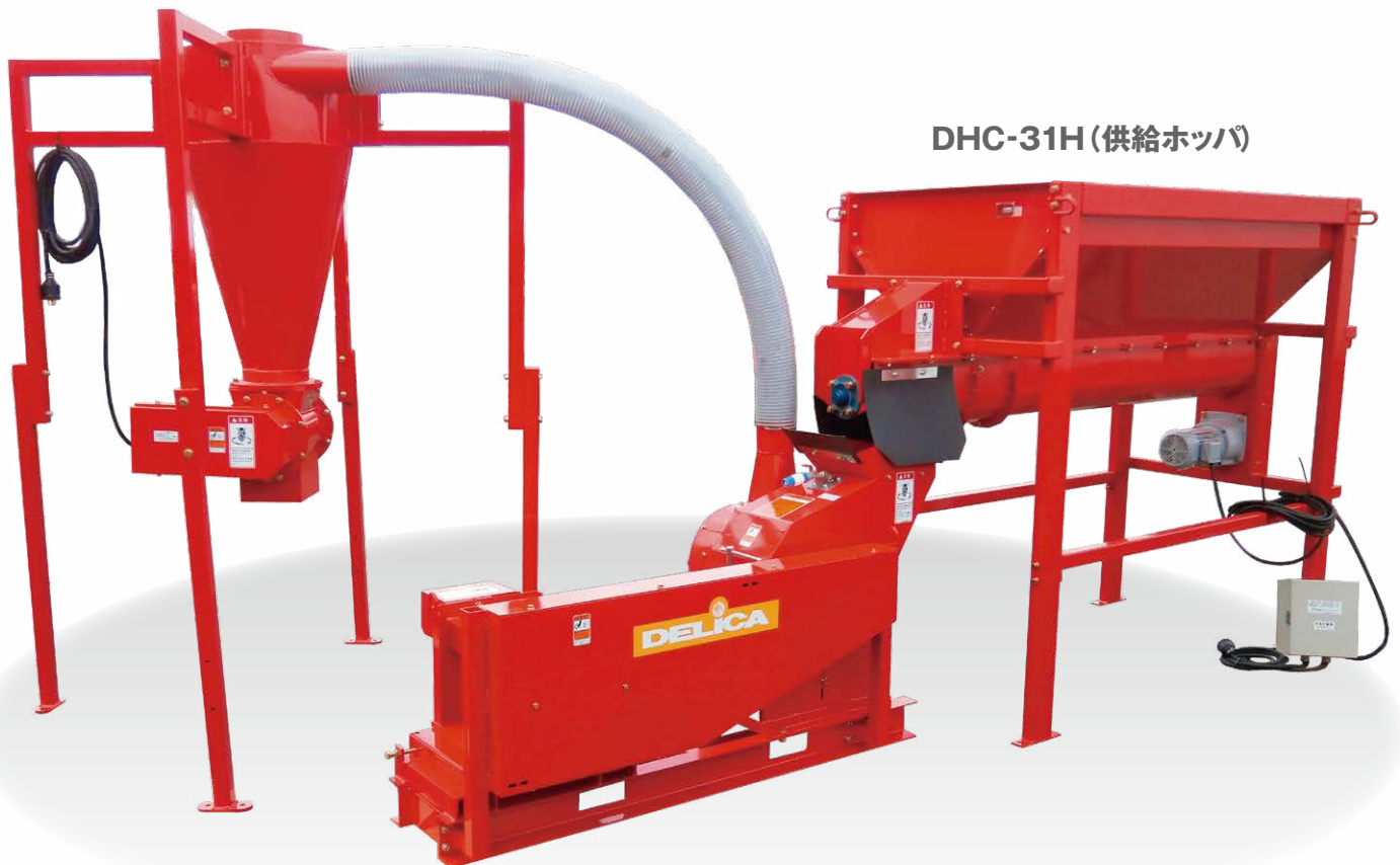
DHC-31T (粉砕機)
